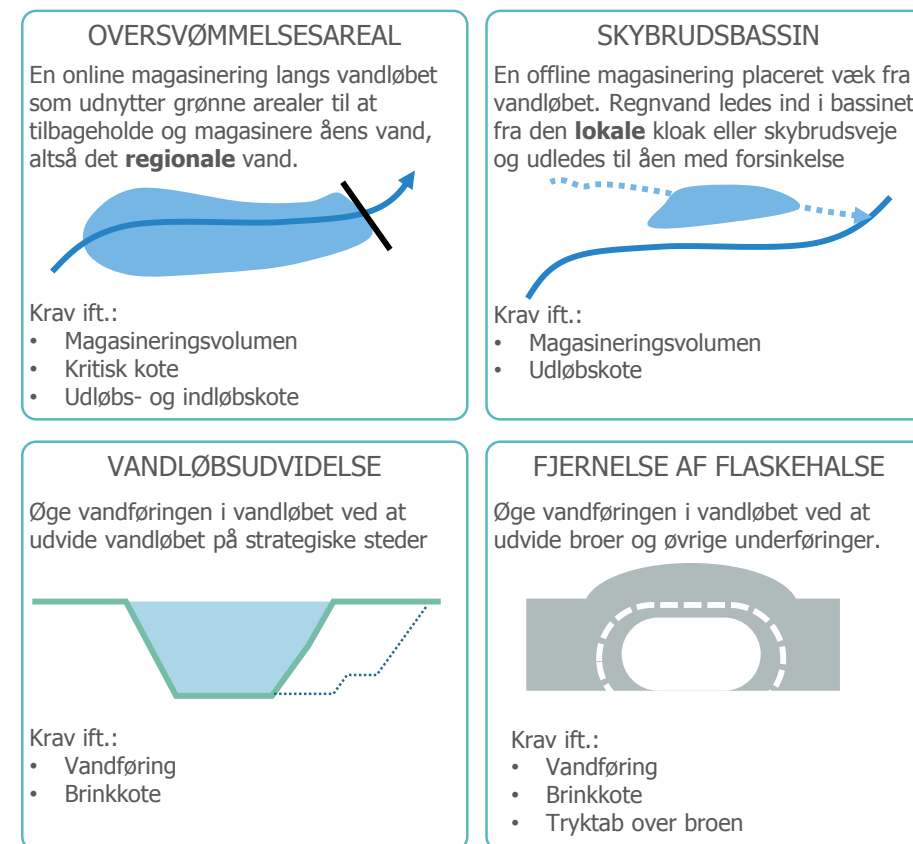
Figur 10. Anlægstyper i Kapacitetsplan 2018. Kravene til hydraulisk funktion er beskrevet i Fagmanualen.
